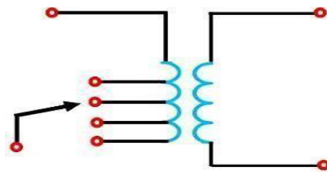
Off-load tap-changing transformer © 2012 M. S. S. S.
