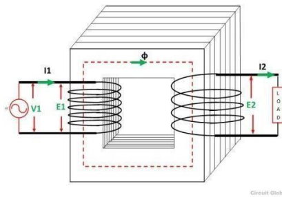
Fig: Simple Transformer
